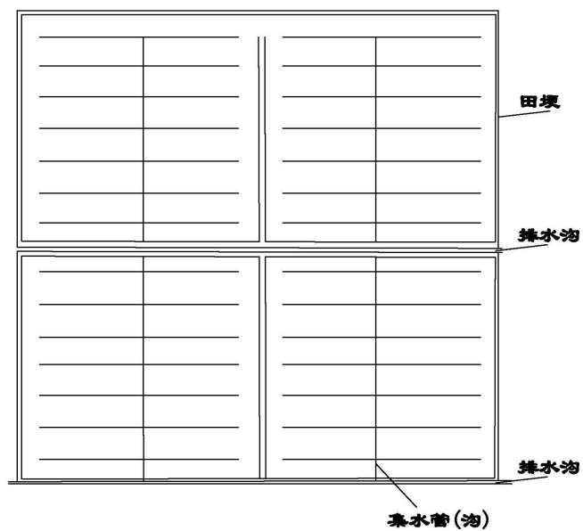
暗管布置方式图
